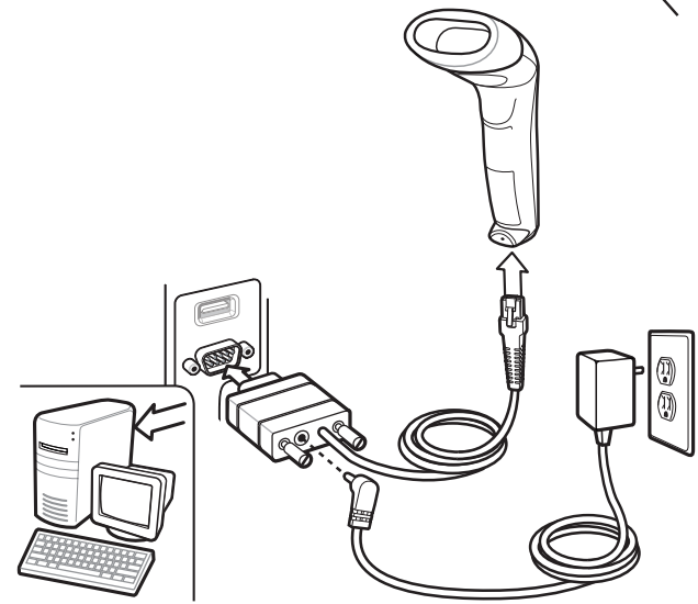
RS-232
